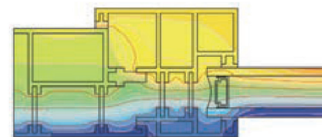
Schéma isothermique de l'intercalaire Warm Edge
