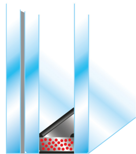
44.2/16/4 (Reconnu par les assurances) (coef Ug=1,1) (Rw 33db)
