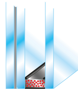
SP 10/16/4 (Reconnu par les assurances) (coef Ug=1,1) (Rw 34db)
