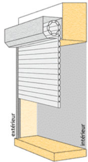
Pose en applique enroulement extérieur
