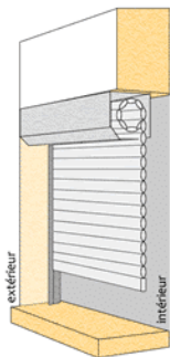
Pose en tableau enroulement extérieur ou inter
