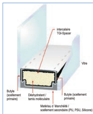
Coupe de interalie Warm Edge
